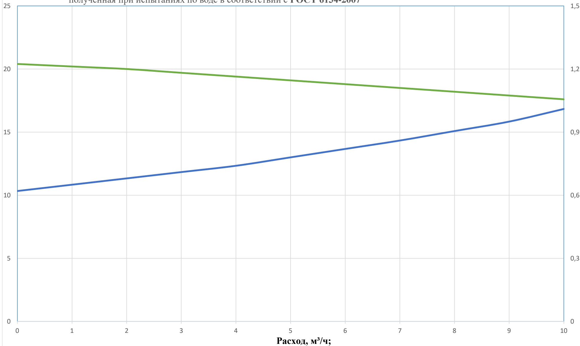
Напорно-энергетическая характеристика ОНЦ 3,5/20К5-1,1/2 с открытым рабочим колесом Ø118мм. полученная при испытаниях по воде в соответствии с ГОСТ 6134-2007
